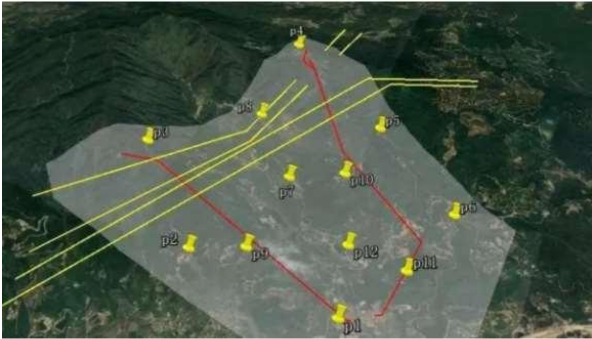
图 4-6 地质监测无人机场景布置及航线规划示意图
