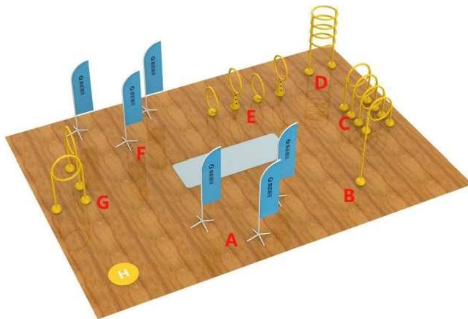
图 4-1 赛道图示
